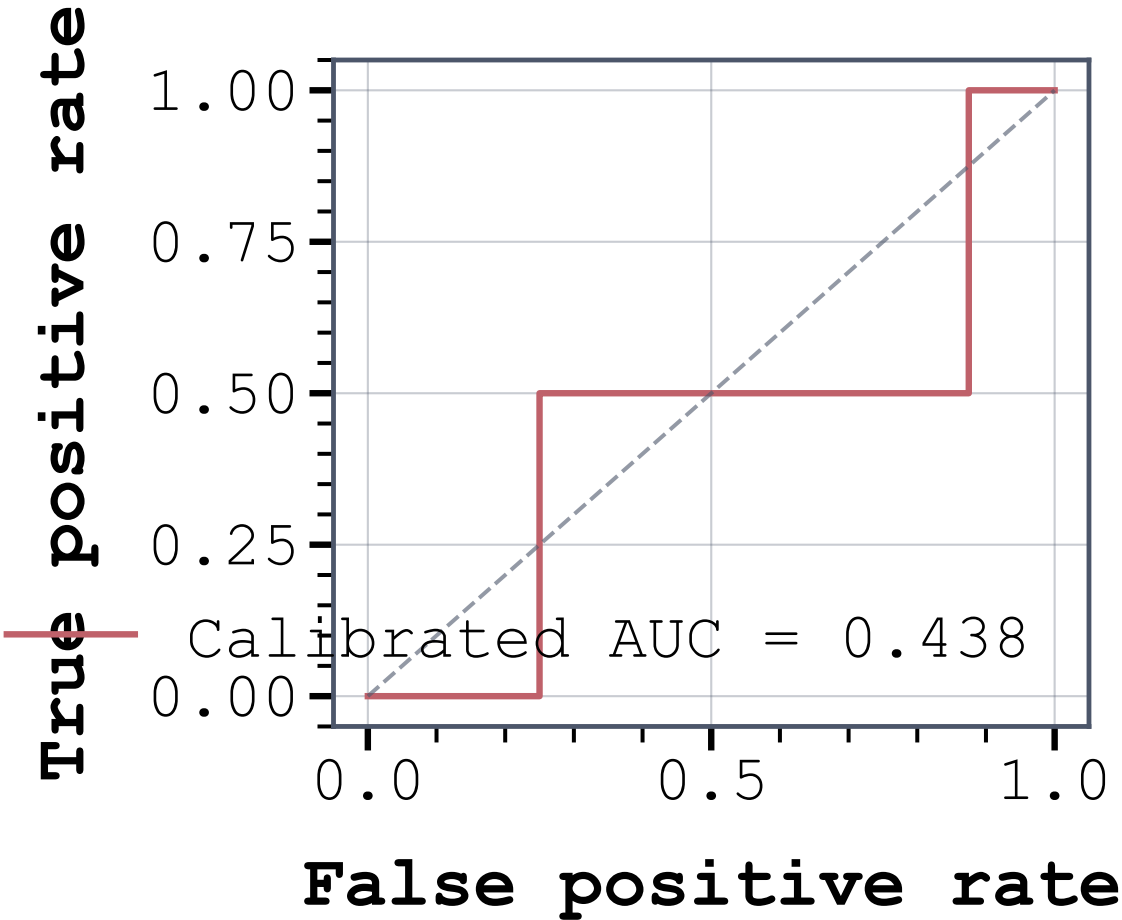
DISPAIR-FRS ROC curveDISPAIR-FRS calibrationDISPAIR-FRS probability distribution
